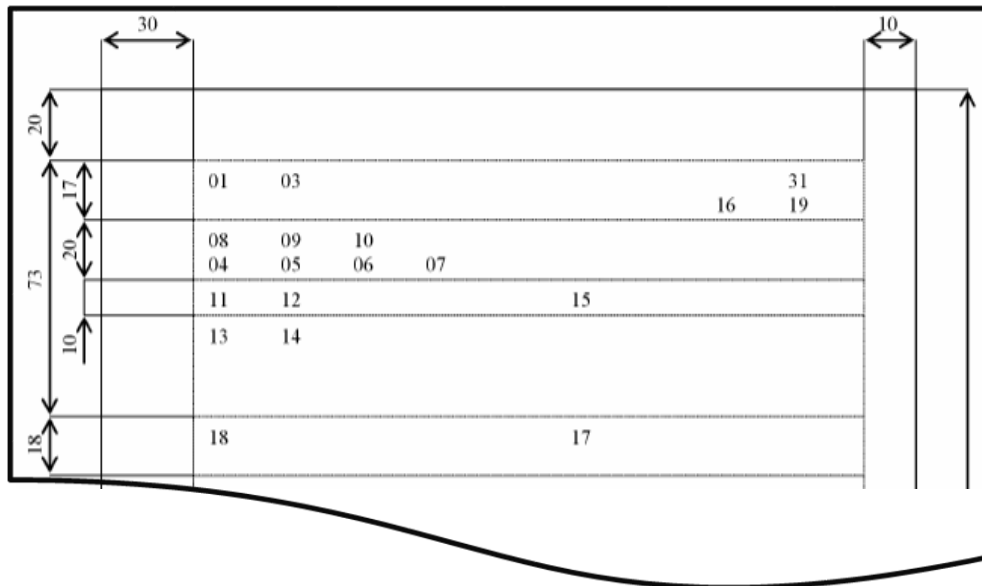
Рис. 2. Расположение реквизитов (продольный вариант) бланка письма (размеры указаны в миллиметрах)
